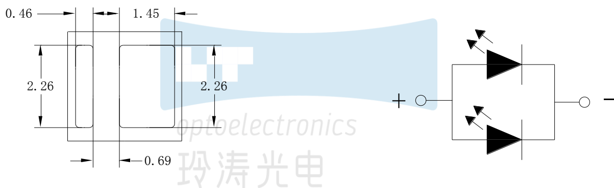
Fig.1-3 Bottom view 背面视图
