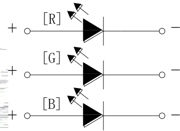
Fig.1-4 Polarity 极性
