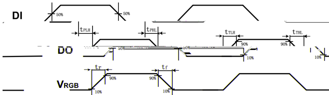
Fig.1-15 交流参数示意图
