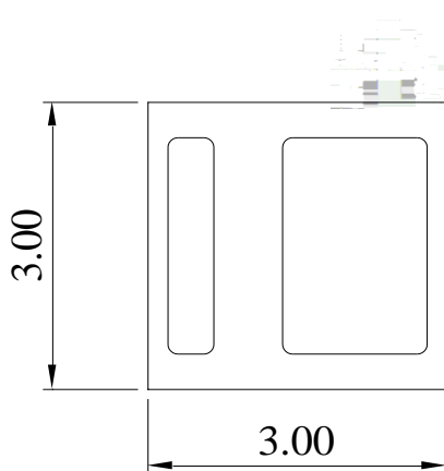
Fig.1-4 Bottom view 背面视图
