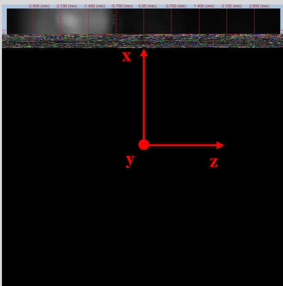
13 I=90^\circ, A=90^\circ
